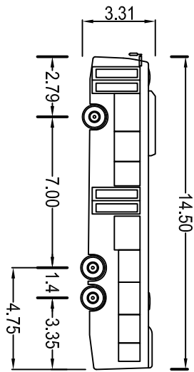
VOLVO B12 BLE (6 x 2)
